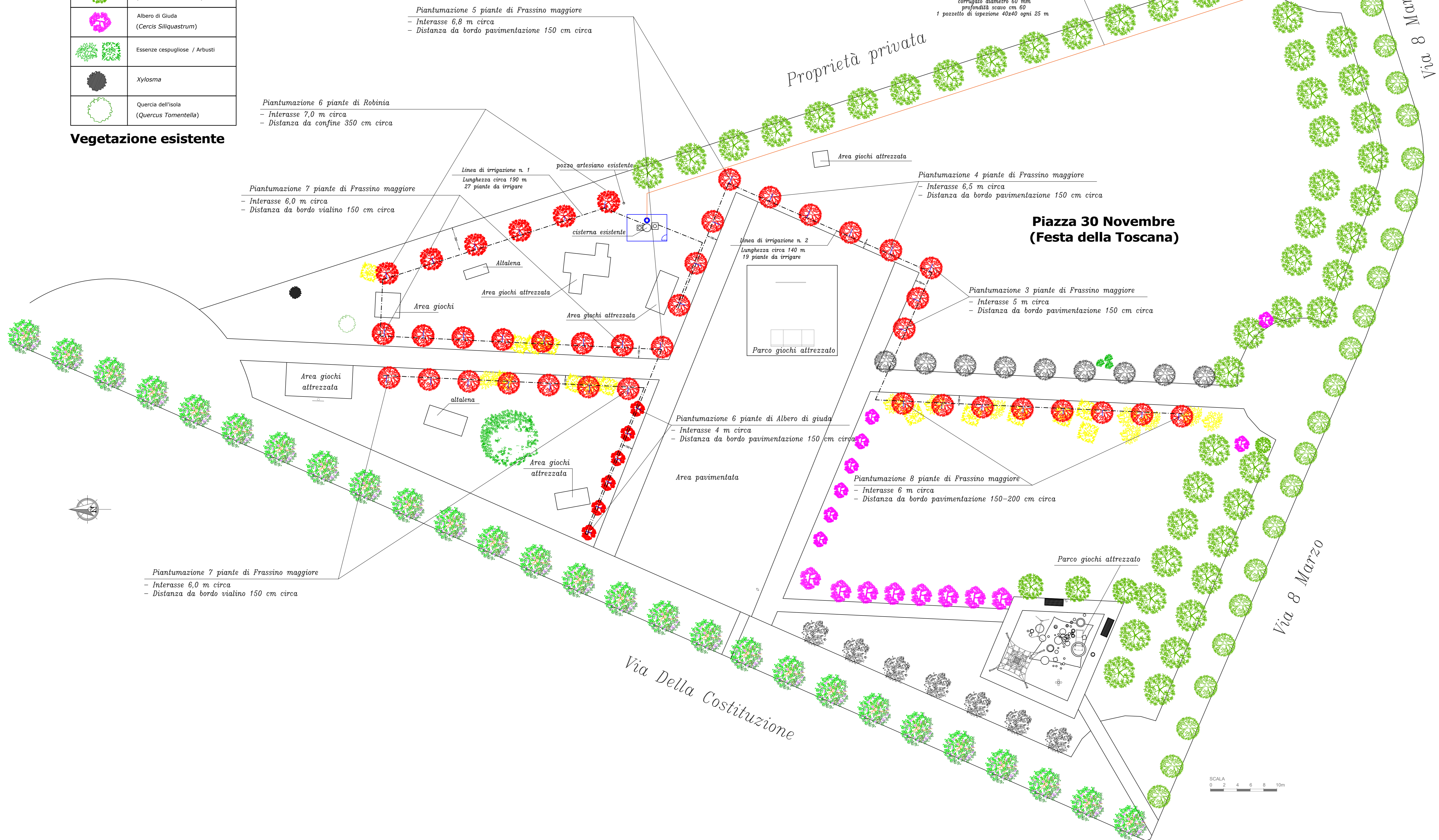
Planimetria generale 1:200
